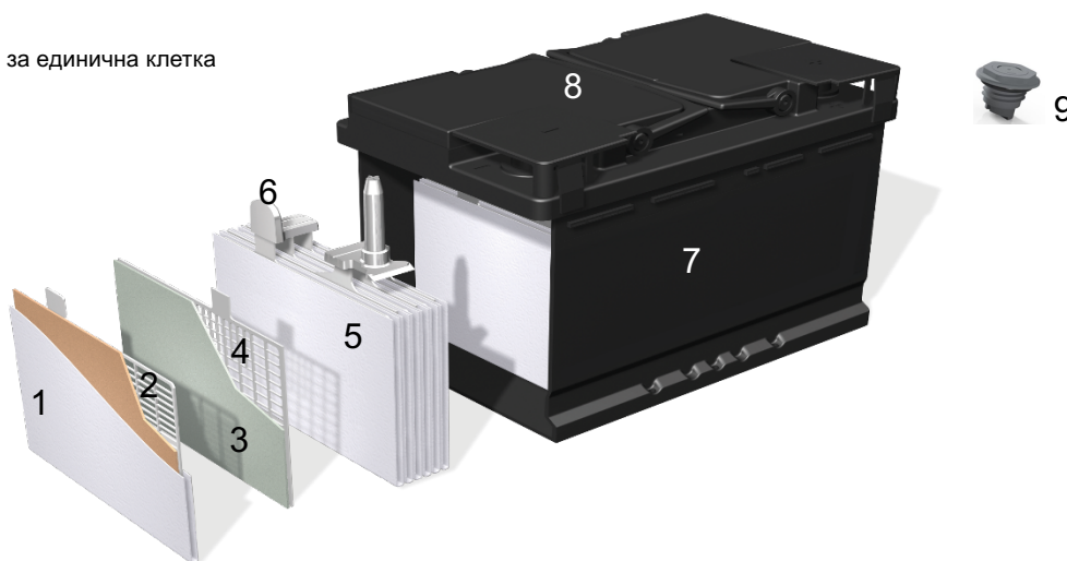
Фигура 1 - Концептуален дизайн на призматична VRLA-AGM оловно-киселинна батерия
