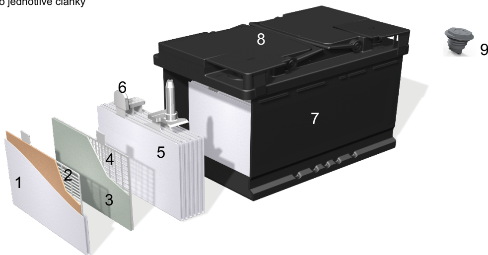
Obrázek 1 – Konceptní návrh konstrukce prizmatické olověné baterie VRLA-AGM
