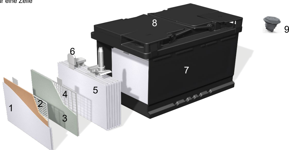
Abbildung 1 – Aufbau einer prismatischen VRLA-AGM-Blei-Säure-Batterie
