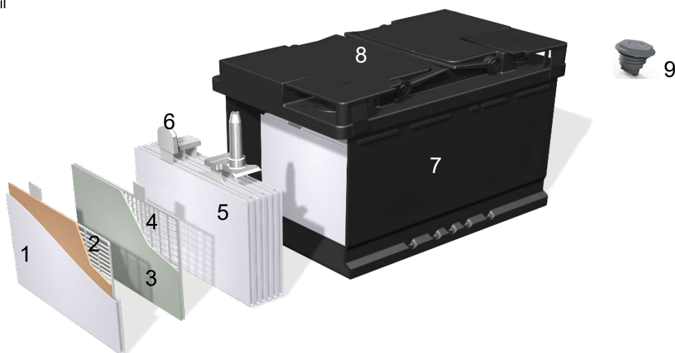
Figur 1 - Konceptuelt design af et prismatisk VRLA-AGM blybatteri
