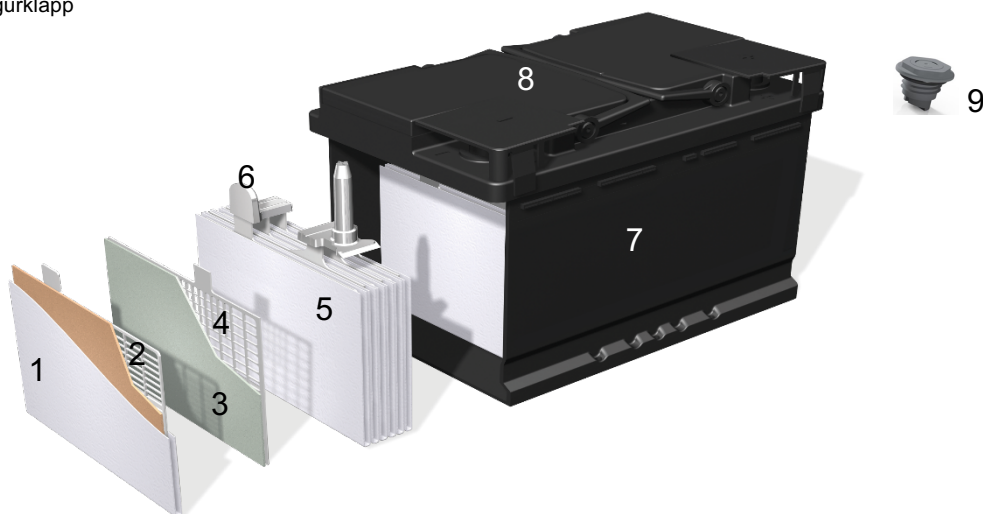
Joonis 1 – Prismaatilise VRLA-AGM pliihappeaku kontseptuaalne disain
