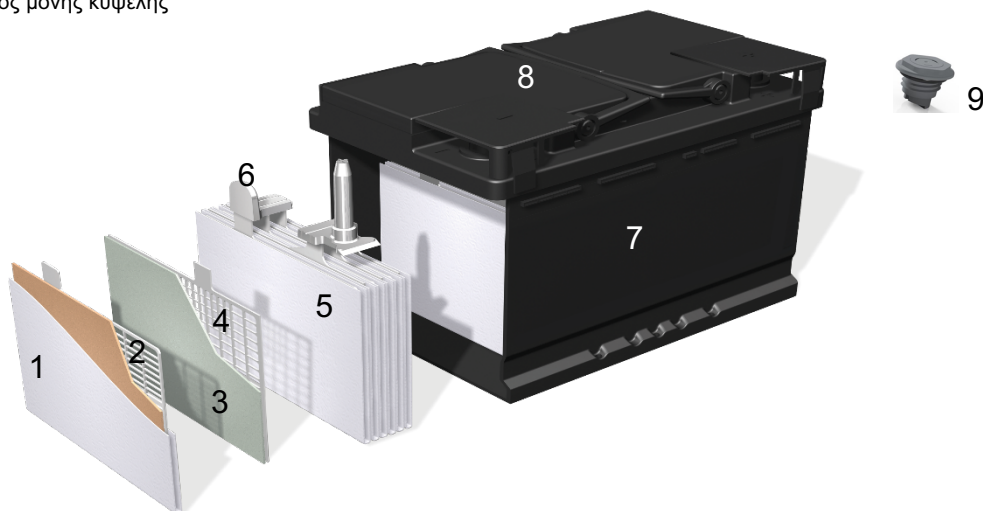
Σχήμα 1 - Εννοιολογικός σχεδιασμός μιας πρισματικής μπαταρίας μολύβδου-οξέος VRLA-AGM
