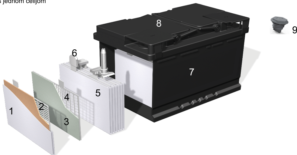
Slika 1. – Koncept dizajna prizmatične olovno-kiselinske baterije VRLA-AGM
