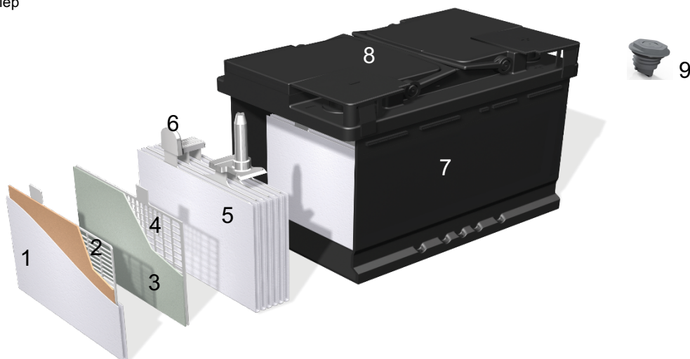
1. ábra – Prizmatikus VRLA-AGM típusú ólom-sav akkumulátor koncepcionális terve
