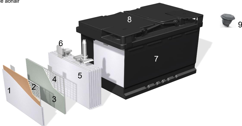
Fíor 1-dearadh Coincheapúil ceallraí aigéad luaidhe vrla-CGB príosmach
