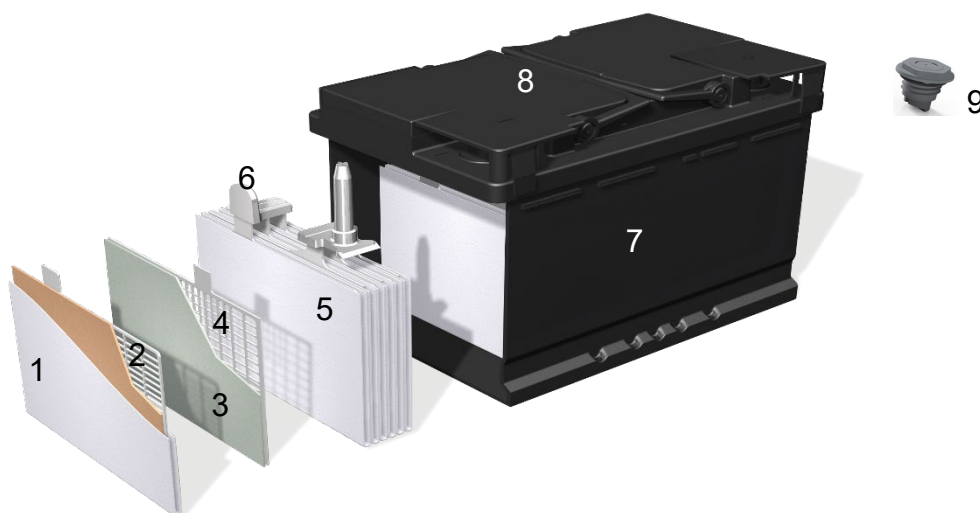
Figura 1 - Progetto concettuale di una batteria prismatica al piombo VRLA-AGM
