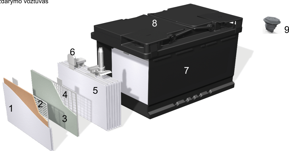
1 iliustracija. VRLA-AGM švino rūgšties akumuliatoriaus koncepcinis dizainas
