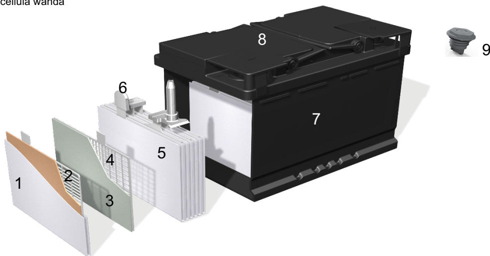
Figura 1 - Disinn kunċettwali ta' batterija prizmatika tač-čomb u l-ačidu VRLA-AGM
