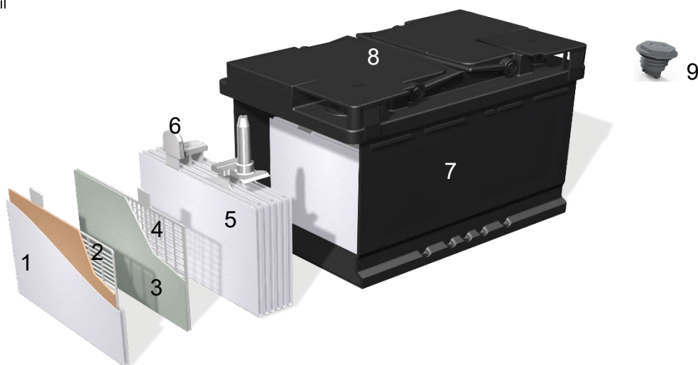
Figur 1 – Konseptuell design av et prismatisk VRLA-AGM blybatteri
