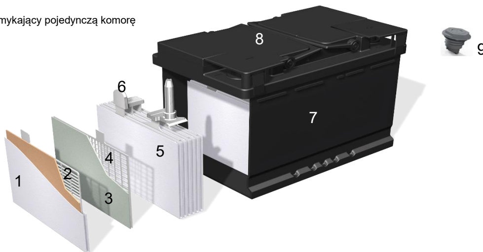
Schemat 1 – projekt koncepcyjny akumulatora kwasowo-ołowiowego VRLA-AGM
