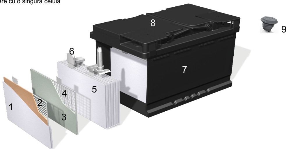
Figura 1-proiectarea conceptuală a unei baterii prismatice cu plumb acid VRLA-AGM
