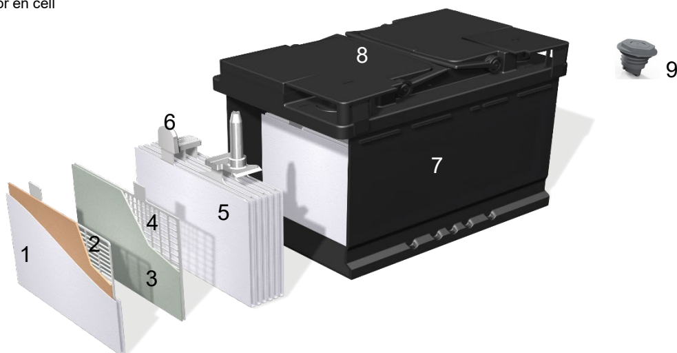
Figur 1 - Konceptuell design av ett prismatiskt VRLA-AGM blybatteri
