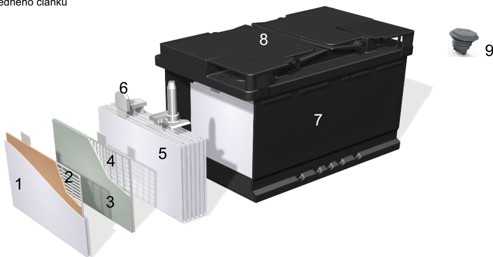
Obrázok 1 – Konceptný návrh prizmatickej oloveno-kyselinovej batérie VRLA-AGM
