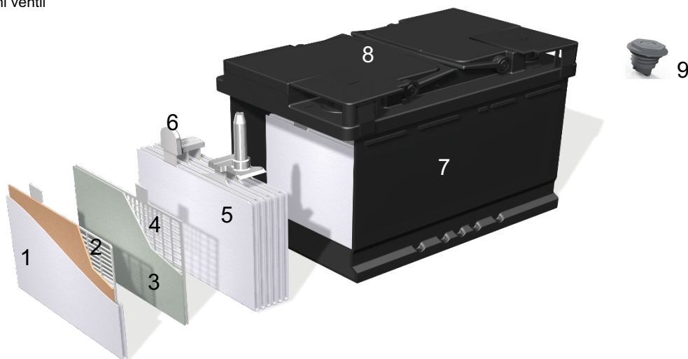
Slika 1 – idejna zasnova prizmatičnega svinčevega akumulatorja VRLA-AGM
