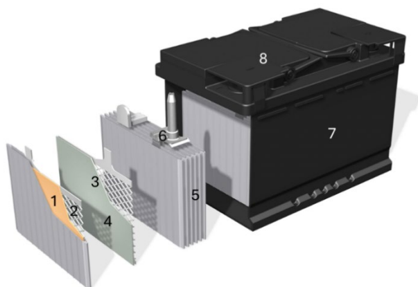
Abbildung 1 – Aufbau einer Blei-Säure-Nassbatterie für Leichtfahrzeuge
