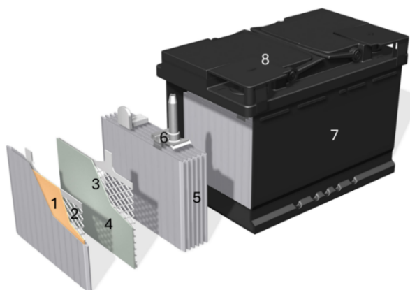
1. ábra – Személygépjárművekhez használható folyadékos típusú ólom-sav akkumulátor koncepcionális terve
