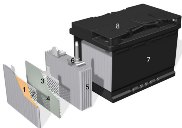
Fíor 1 – Dearadh coincheapúil ceallraí aigéad luaidhe LV faoi thuilte
