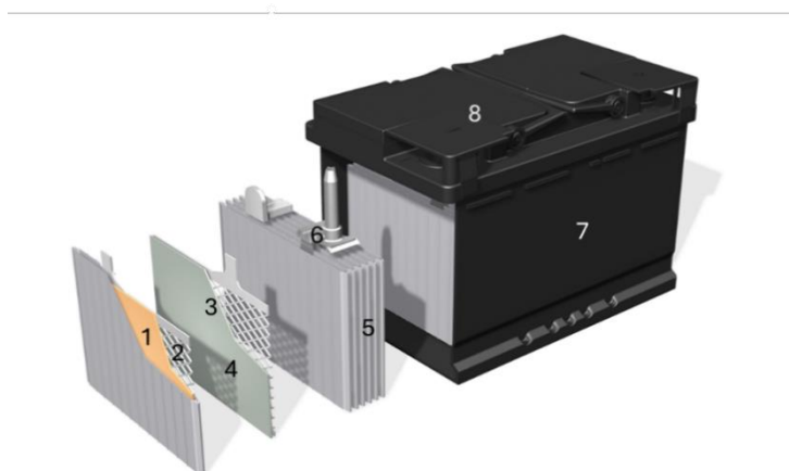
Schemat 1 – Projekt koncepcyjny kwasowo-ołowiowego zalewanego akumulatora do pojazdów osobowych
