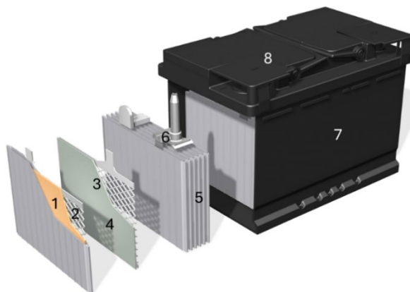
Figur 1 – Konceptuell design av ett LV Flooded blybatteri
