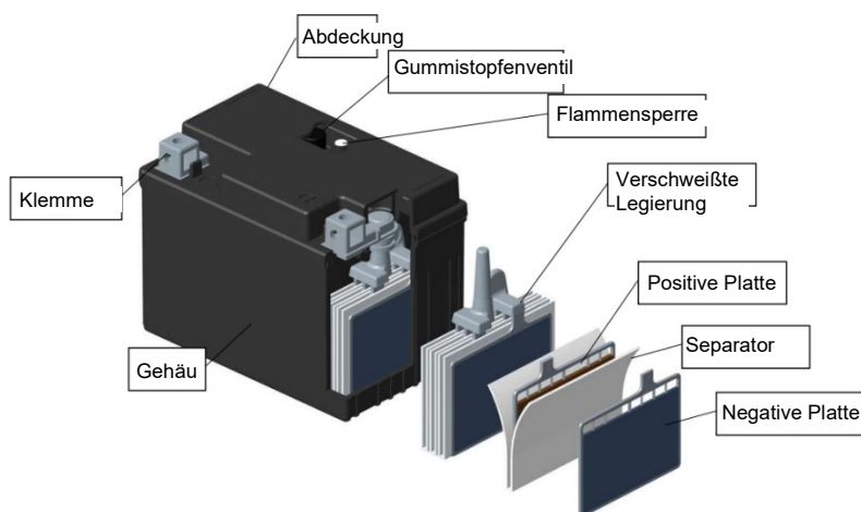
Abbildung 1 – Aufbau einer VRLA-AGM-Blei-Säure-Motorradbatterie
