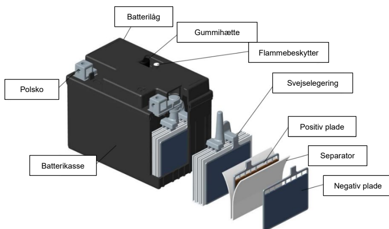
Figur 1 - Konceptuelt design af et MC VRLA-AGM-blybatteri
