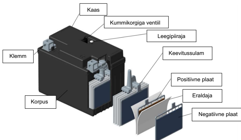
Joonis 1 – Mootorratta VRLA-AGM pliihappeaku kontseptuaalne disain
