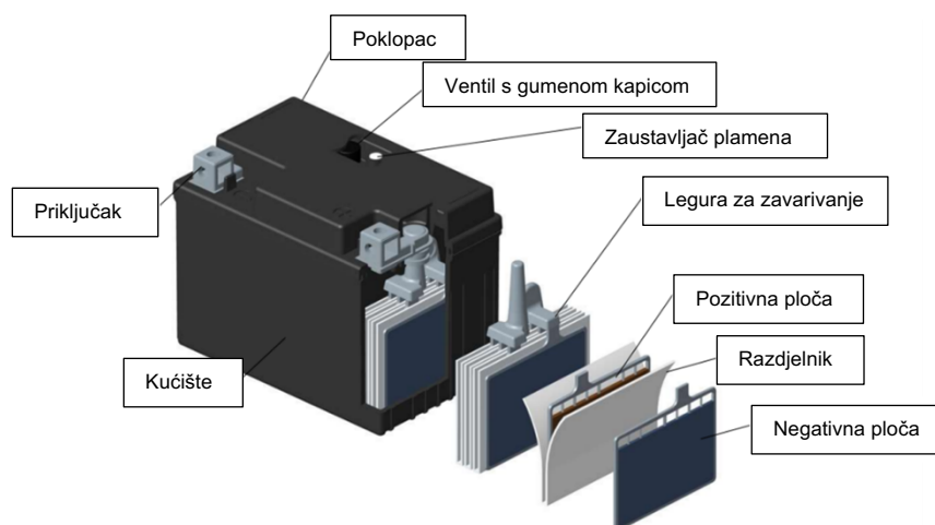
Slika 1. – Koncept dizajna olovno-kiselinske baterije VRLA-AGM za motocikle
