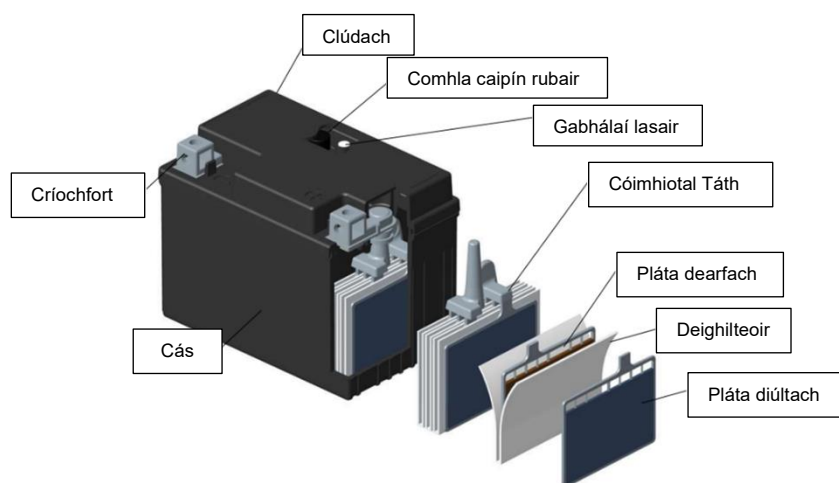
Fíor 1 - Dearadh coincheapúil ceallraí aigéad luaidhe MC VRLA-AGM
