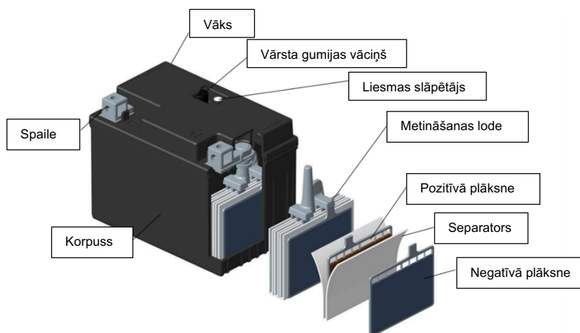
1. attēls. MC VRLA-AGM svina-skābes akumulatora konstrukcijas mets
