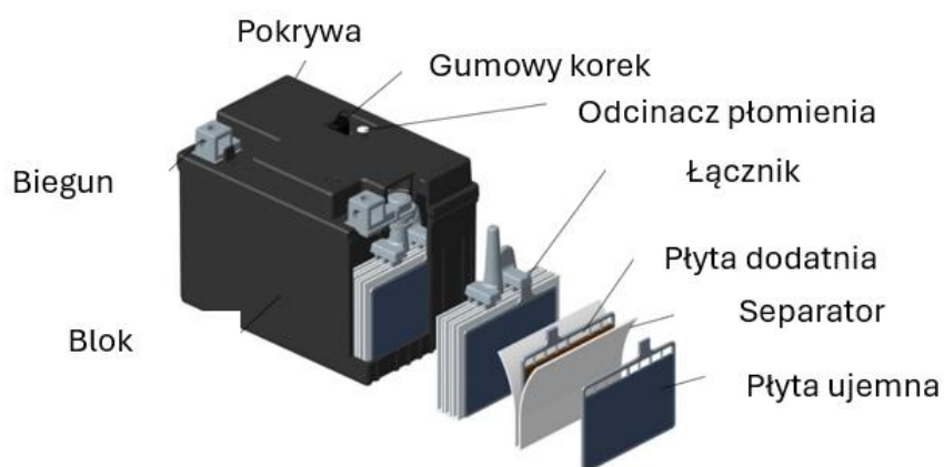
Schemat 1 – Projekt koncepcyjny akumulatora kwasowo-ołowiowego motocyklowego VRLA-AGM
