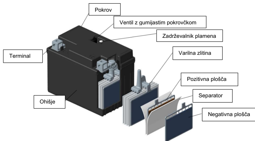
Slika 1 – idejna zasnova svinčevega akumulatorja MC VRLA-AGM
