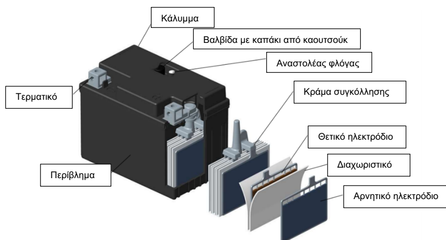
Σχήμα 1 - Εννοιολογικός σχεδιασμός μπαταρίας μολύβδου-οξέος MC VRLA-AGM
