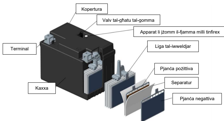
Figura 1 - Disinn kunċettwali ta' batterija taċ-ċomb u l-aċidu MC VRLA-AGM
