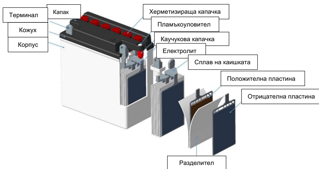
Фигура 1 - Концептуален дизайн на МС наводнена оловно-киселинна батерия
