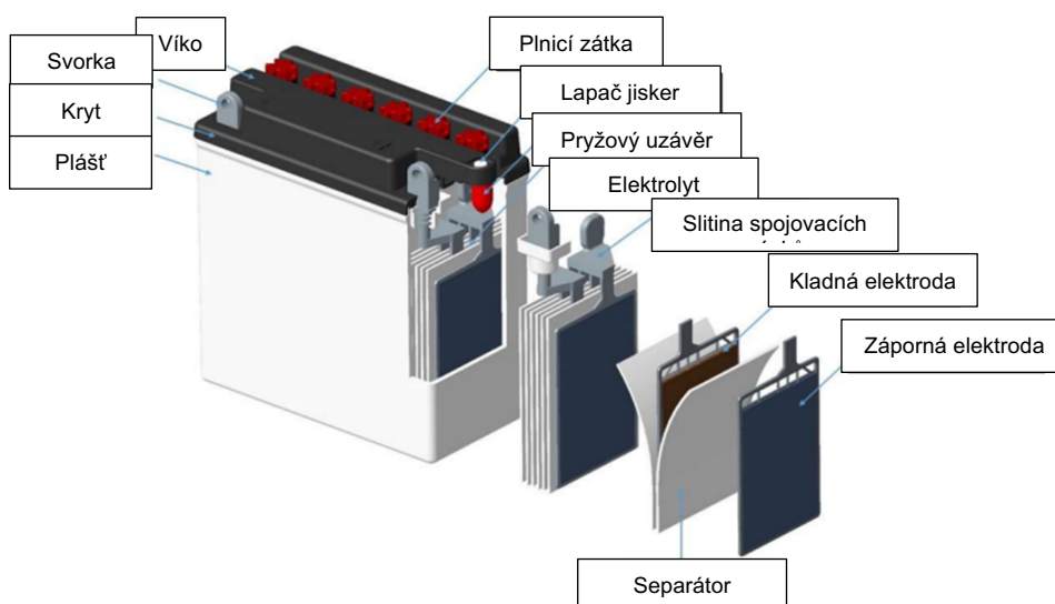
Obrázek 1 – Konceptní návrh konstrukce olověné baterie s kapalným elektrolytem a se středním napětím
