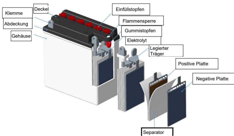
Abbildung 1 – Aufbau einer Blei-Säure-Nassbatterie für Motorräder
