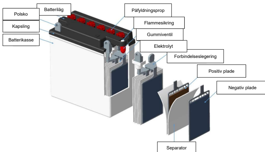
Figur 1 - Konceptuelt design af et MC Flooded blybatteri
