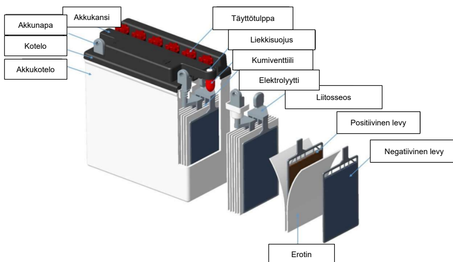
Kuva 1 - MC Flooded -lyijyakun konseptisuunnittelu
