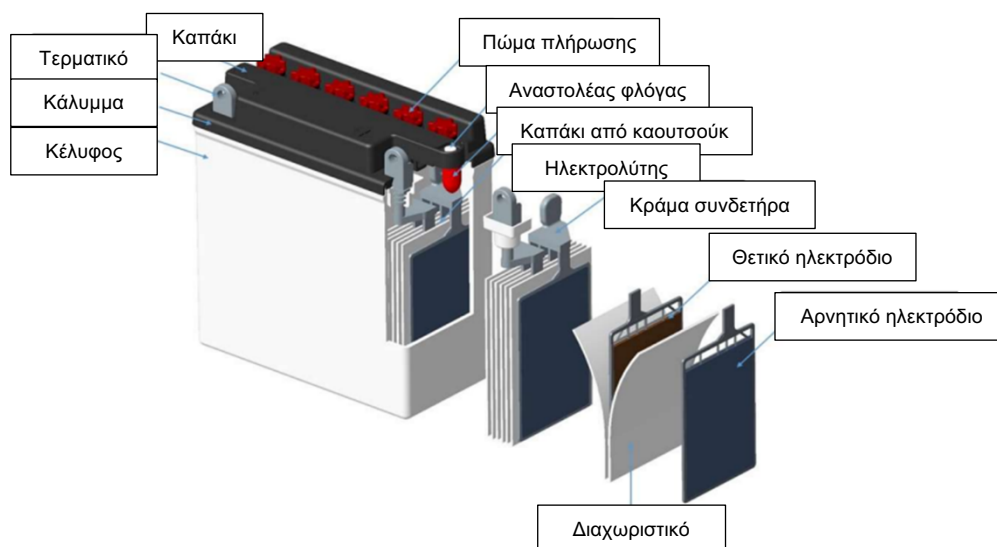
Σχήμα 1 - Εννοιολογικός σχεδιασμός μπαταρίας μολύβδου-οξέος υγρού ηλεκτρολύτη MC
