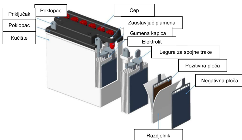
Slika 1. – Koncept dizajna olovno-kiselinske baterije s tekućim elektrolitom za motocikle (MC)
