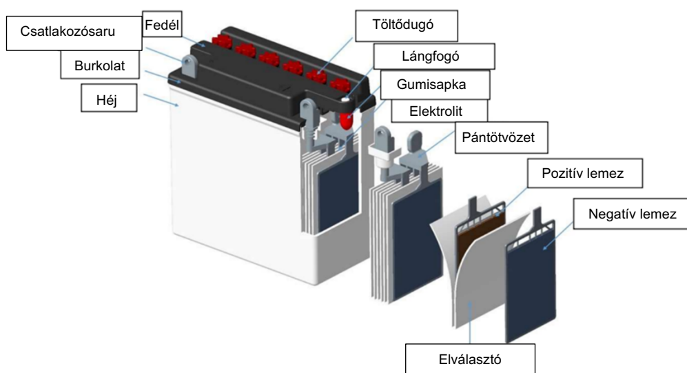
1. ábra – Motorkerékpárokhoz használható folyadékos típusú ólom-sav akkumulátor koncepcionális terve
