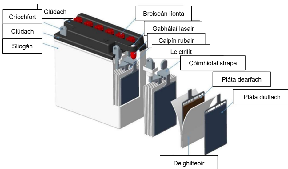
Fíor 1 - Dearadh coincheapúil ceallraí luaidhe-aigéid faoi uisce MC
