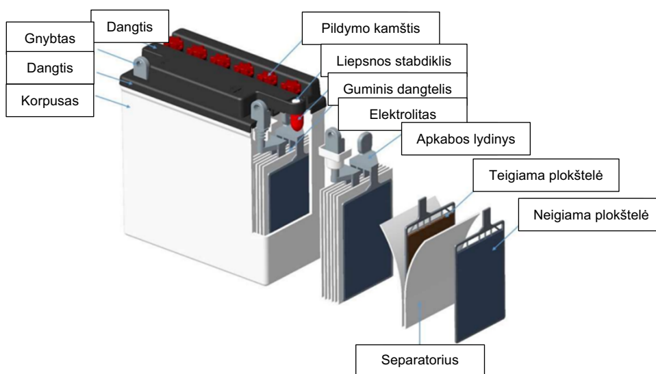
1 iliustracija. MC užtvindyto švino rūgšties akumuliatoriaus koncepcinis dizainas
