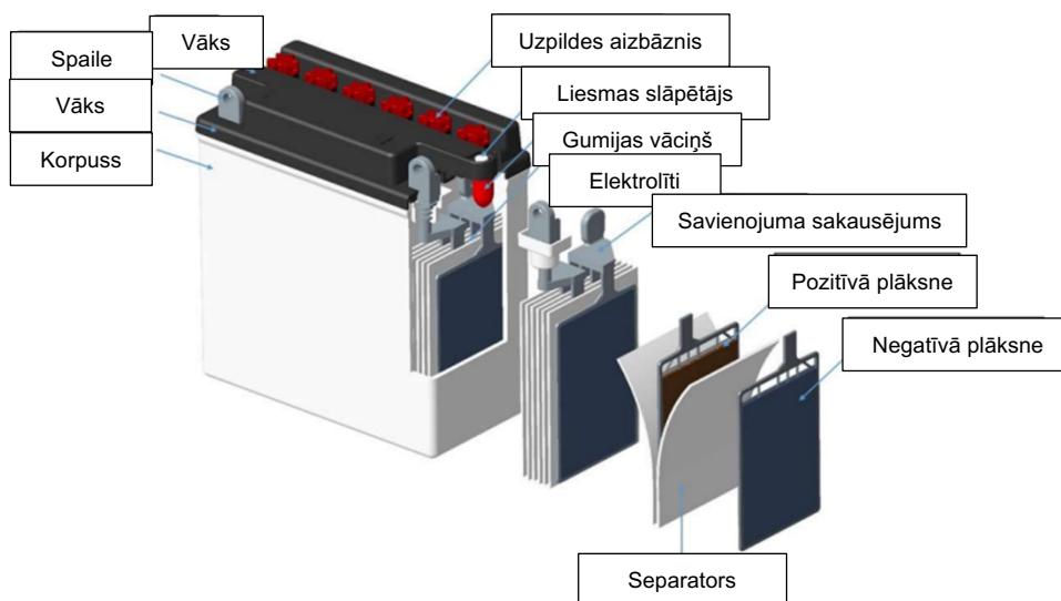
1. attēls. Tehnoloģijas MC Flooded svina-skābes akumulatora konstrukcijas mets
