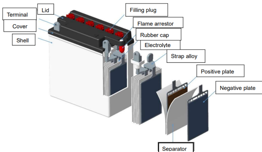
Figuur 1 - Conceptueel ontwerp van een MC Flooded loodzuuraccu
