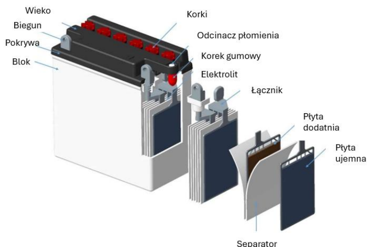
Schemat 1 – Projekt koncepcyjny akumulatora kwasowo-ołowiowego motocyklowego
