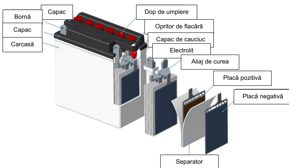
Figura 1 - Proiectarea conceptuală a unei baterii cu plumb acid MC inundată
