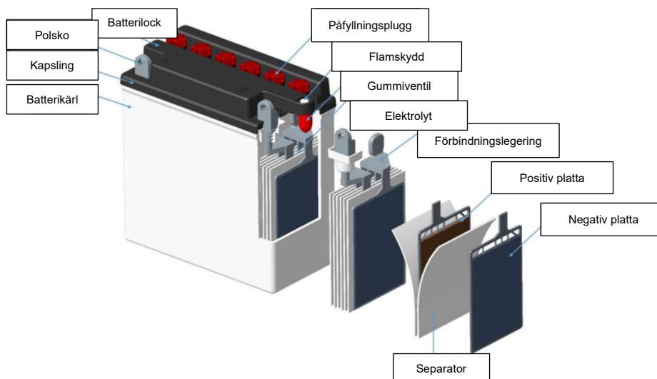
Figur 1 - Konceptuell design av ett MC Flooded blybatteri
