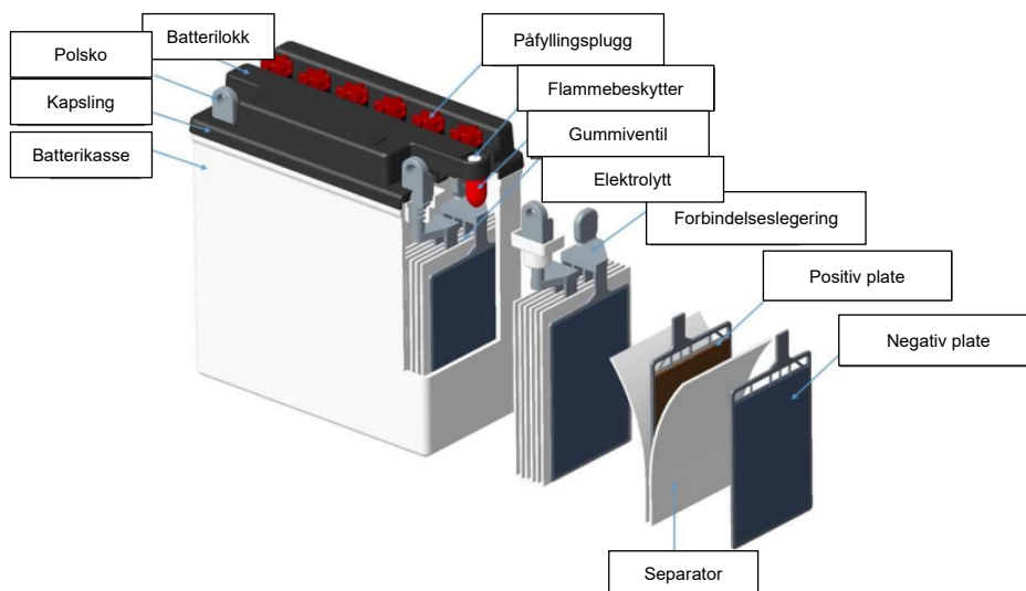
Figur 1 – Konseptuell design av et MC Flooded blybatteri
