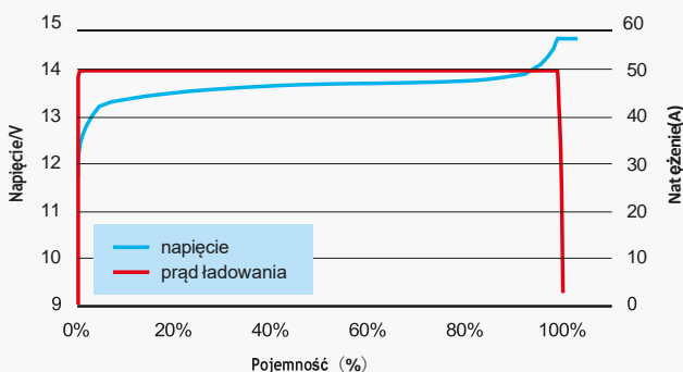
12V100Ah Charakterystyka ładowania 0.5C @RT
