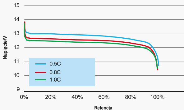
12V100Ah Krzywe rozładowania przy różnych C @RT
